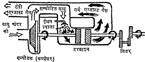
गैसोलीन टरबाइन
