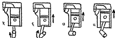
जोड़क डंडा
